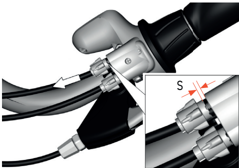
Afbeelding 40: Kabelspeling controleren
