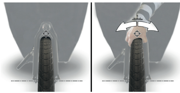
Abbildung 35: Prüfen des Spiels an der Nabenachse
