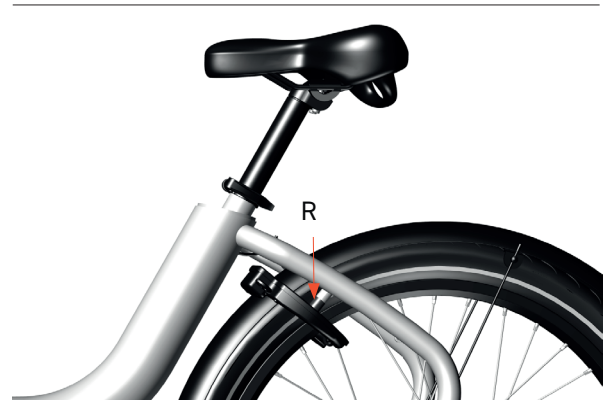
Abbildung 37: Überprüfen der Schlossgummis
