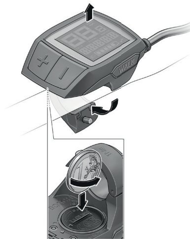
Image 31 : Changer les piles de l'affichage Purion
