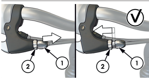
Abbildung 38: Einstellung der Bremszuglänge
