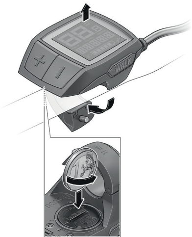
Afbeelding 31: De batterijen van het Purion display vervangen
