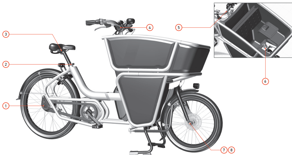
Afbeelding 42: Aandraaimomenten
