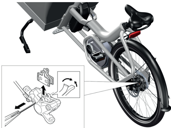
Abbildung 39: Entfernen der Bremsbeläge, um sie auf Verschleiß zu prüfen
