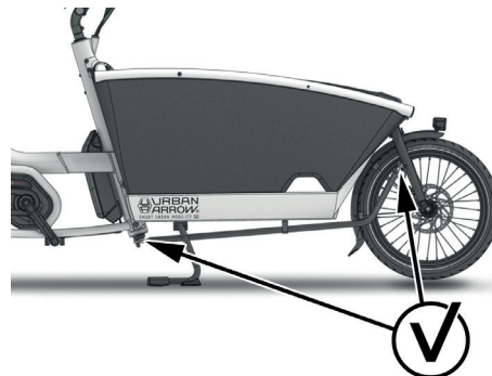
Image 39 : Vérifiez la liaison de la direction au niveau des rotules.
