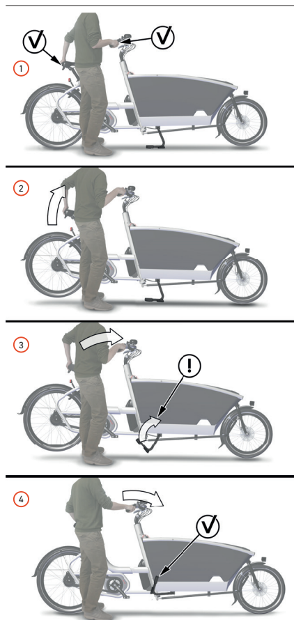
Image 26 : Enlever le vélo de sa béquille
