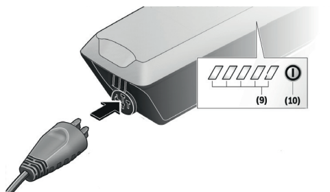
Image 33 : Brancher le connecteur de charge dans la prise de charge de la batterie
