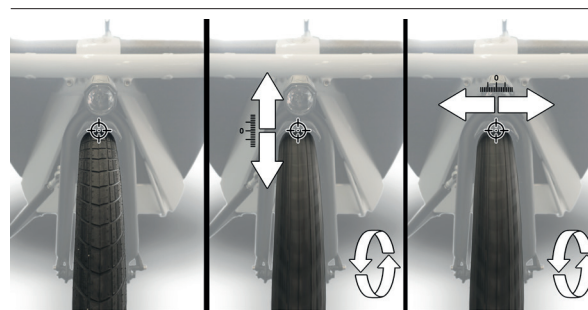
Image 37 : Vérification du décalage de la roue
