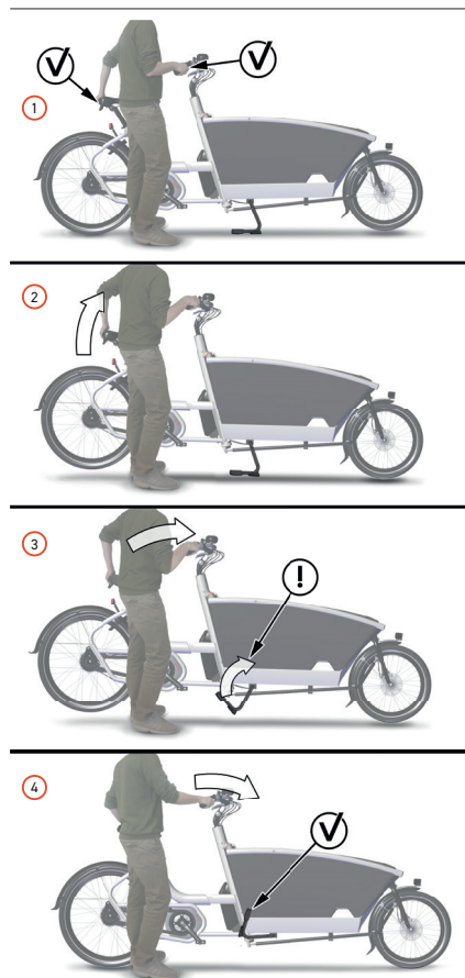
Abbildung 26: Einklappen des Fahrradständers
