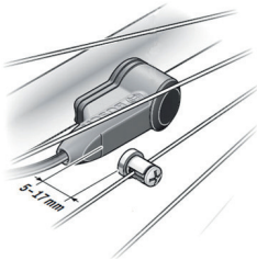
Abbildung 35: Abstand zwischen dem Geschwindigkeitssensor und dem Geschwindigkeitssensormagneten
