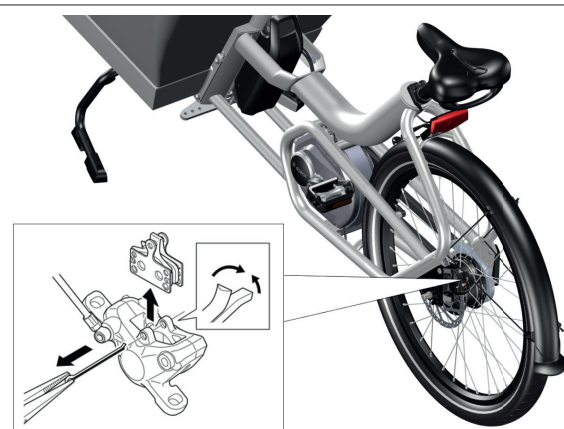
Abbildung 42: Entfernen der Bremsbeläge, um sie auf Verschleiß zu prüfen
