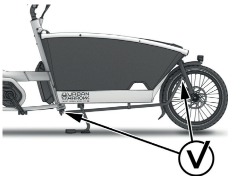
Afbeelding 39: Controleer de stuuroverbrenging bij de kogelgewrichten
