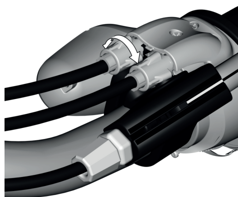
Abbildung 44: Reduzierung oder Erhöhung des Kabelspiels durch Drehen der Zugeinstellschraube am Griffschalter
