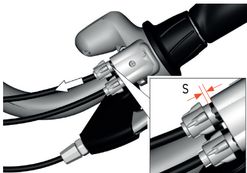
Abbildung 43: Kontrolle des Kabelspiels
