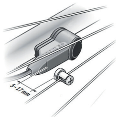
Afbeelding 35: Afstand tussen de snelheidssensor en de magneet van de snelheidssensor
