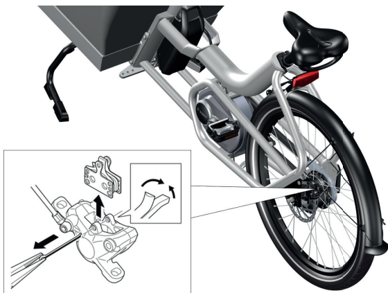
Image 42 : Retrait des plaquettes de frein afin de vérifier leur état d'usure
