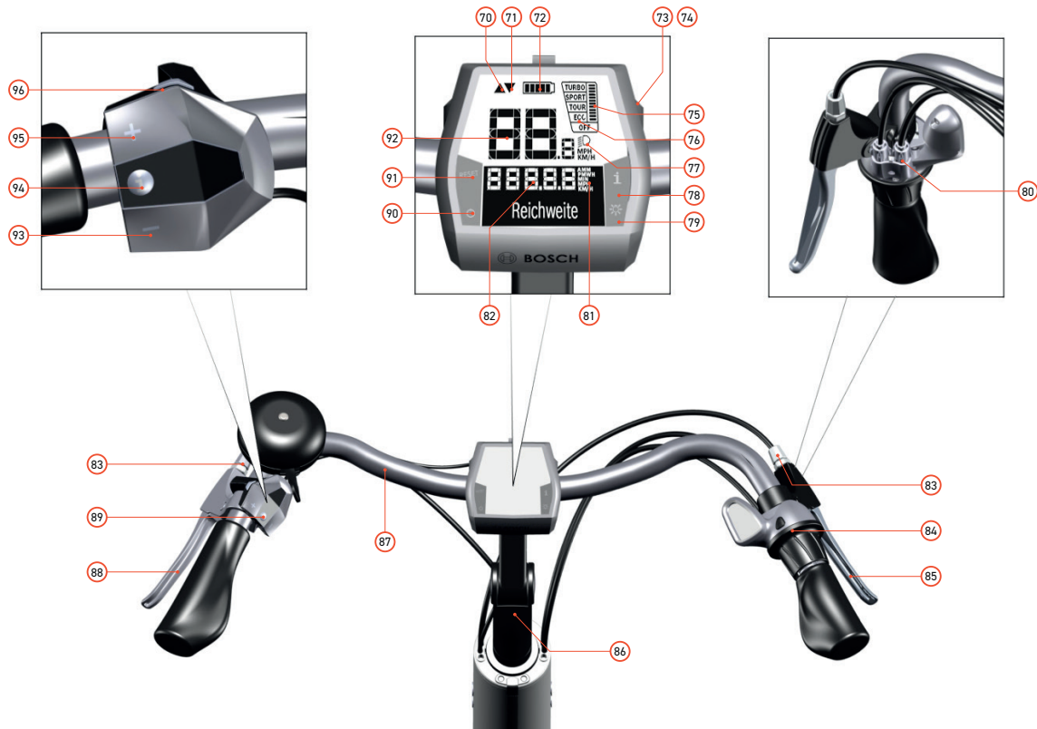
Afbeelding 3: Stuur met Intuvia display en versnellingspook met versnellingsindicator
