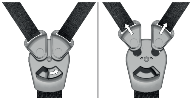
Abbildung 23: Öffnen des Sicherheitsgurts
