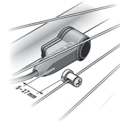
Image 35 : Distance entre le capteur de vitesse et l'aimant de rayon du capteur de vitesse
