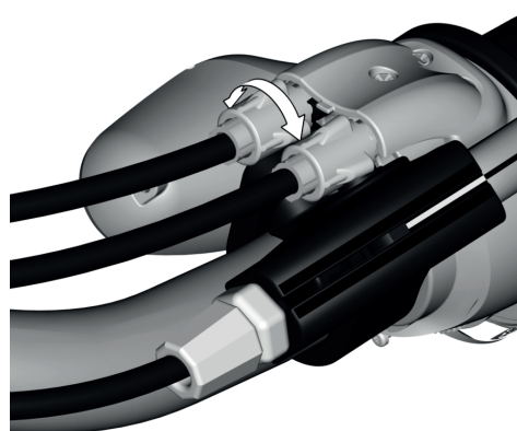
Afbeelding 44: Verminderen of vergroten van de speling van de kabel door de bus aan de draaiversteller te draaien
