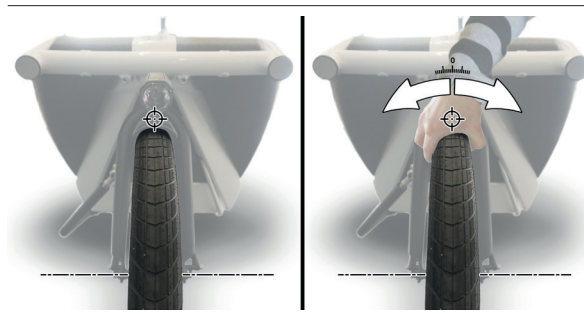
Abbildung 38: Prüfen des Spiels an der Nabenachse
