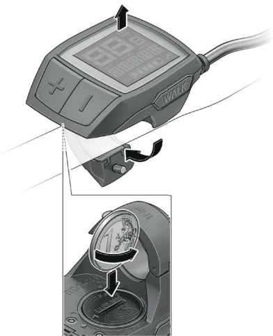
Afbeelding 34: De batterijen van het Purion display vervangen
