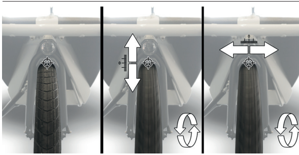
Afbeelding 37: De centrering van het wiel controleren
