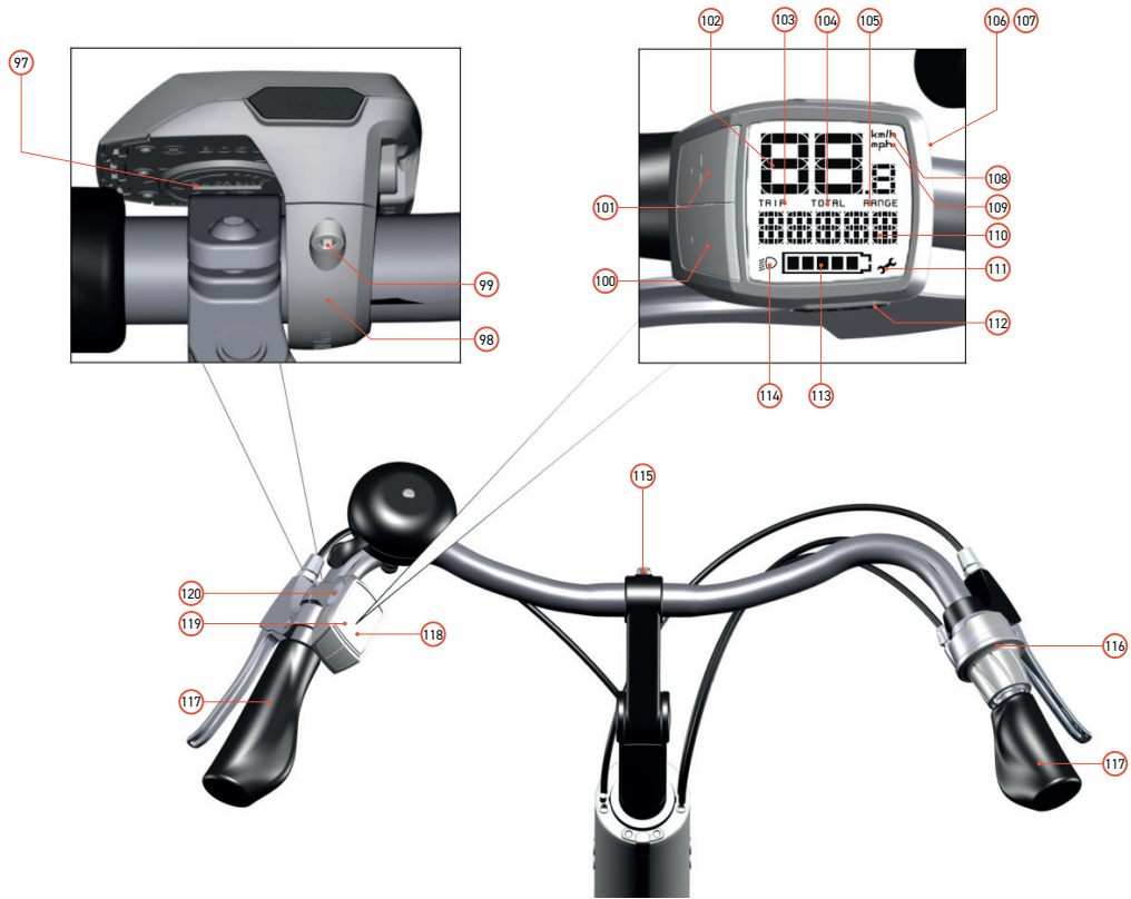
Afbeelding 4: Stuur met Purion display en versnellingspook zonder versnellingsindicator
