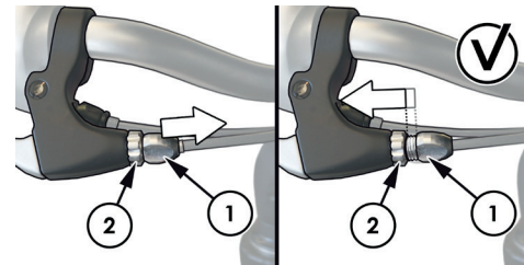
Abbildung 41: Einstellung der Bremszuglänge
