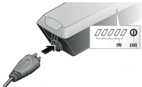
Abbildung 33: Ladegerätstecker in die Ladebuchse am Akku stecken.
