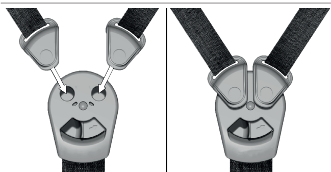
Image 22 : Fermer le harnais de sécurité
