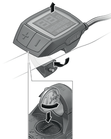
Image 34 : Changer les piles de l'affichage Purion
