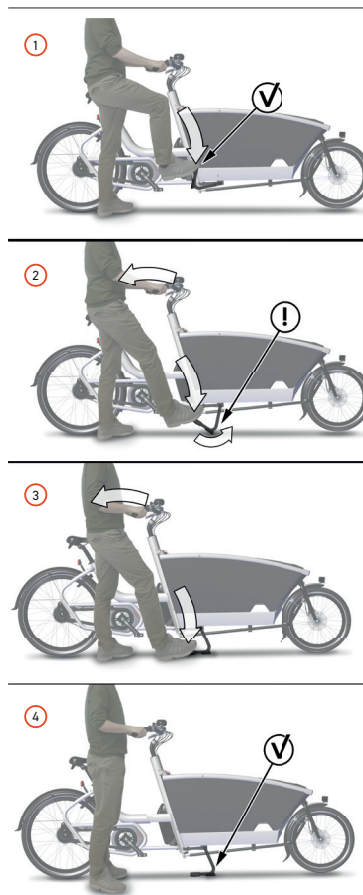
Image 25 : Mettre le vélo sur sa béquille
