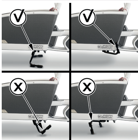
Image 27 : Positions correctes et incorrectes de la béquille
