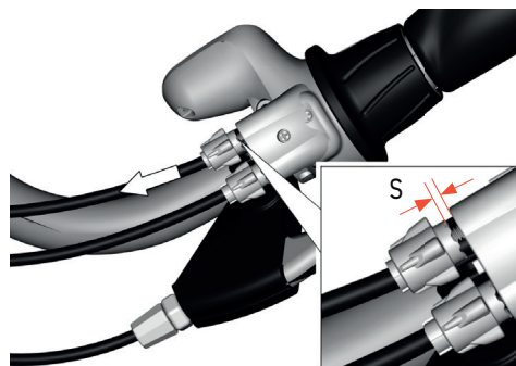
Image 43 : Vérification du jeu du câble
