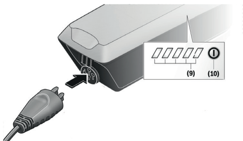
Afbeelding 33: Steek de laadstekker in de laadaansluiting op de accu
