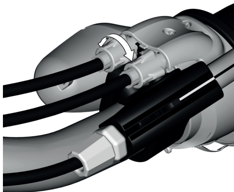
Image 44 : Réduire ou augmenter le jeu du câble en tournant le cylindre sur la poignée de changement de vitesses
