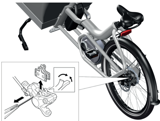
Afbeelding 42: Verwijderen van de remblokjes om ze op slijtage te controleren
