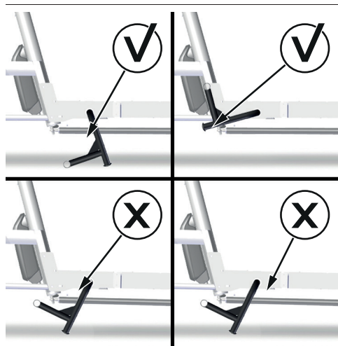
Afbeelding 24: Correcte en onjuiste standen van de standaard
