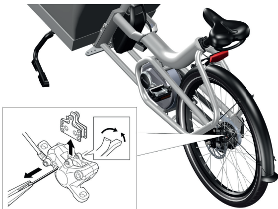
Afbeelding 38: Verwijderen van de remblokken om ze op slijtage te controleren
