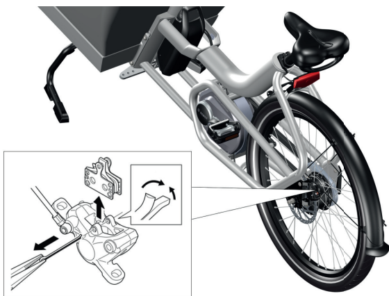
Abbildung 38: Entfernen der Bremsbeläge, um sie auf Verschleiß zu prüfen
